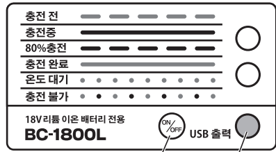
USB출력 스위치
