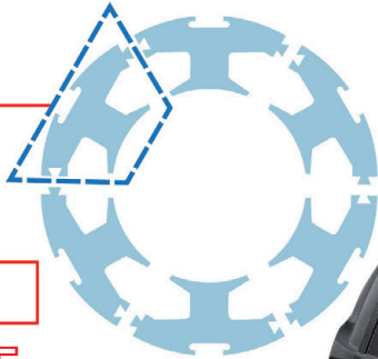
[브러시 리스 분할 모터 단면도]
